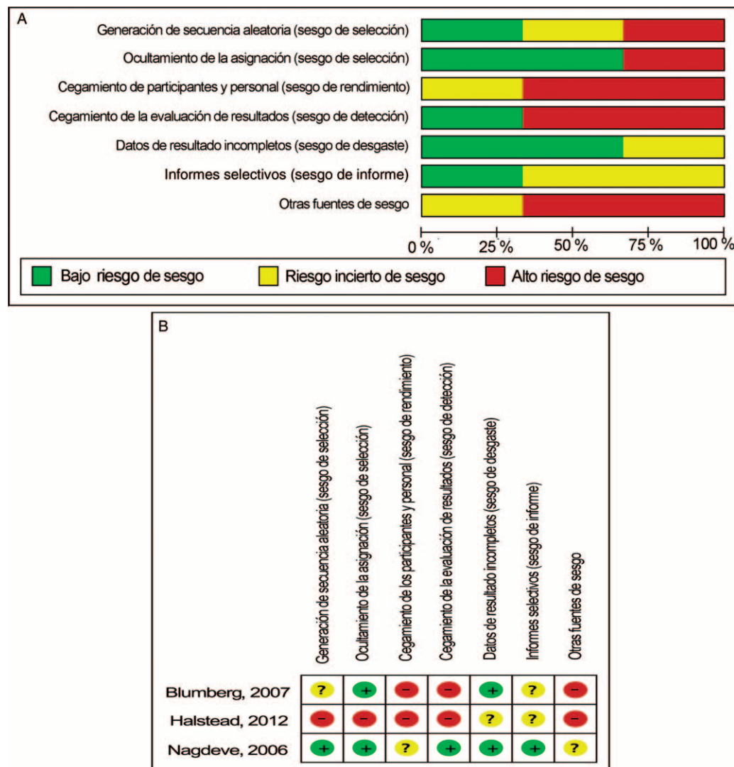
Figura 2. (a and b) Evaluación de riesgo de sesgo de estudios individuales según escala de colaboración Cochrane. Fuente: Autores.
