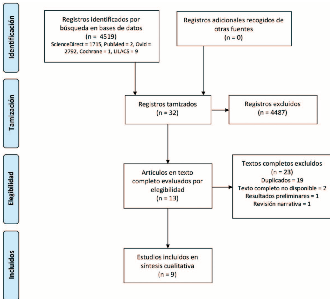
Figura 1. Diagrama de flujo PRISMA que ilustra el proceso de identificación, tamización y selección de estudios.
